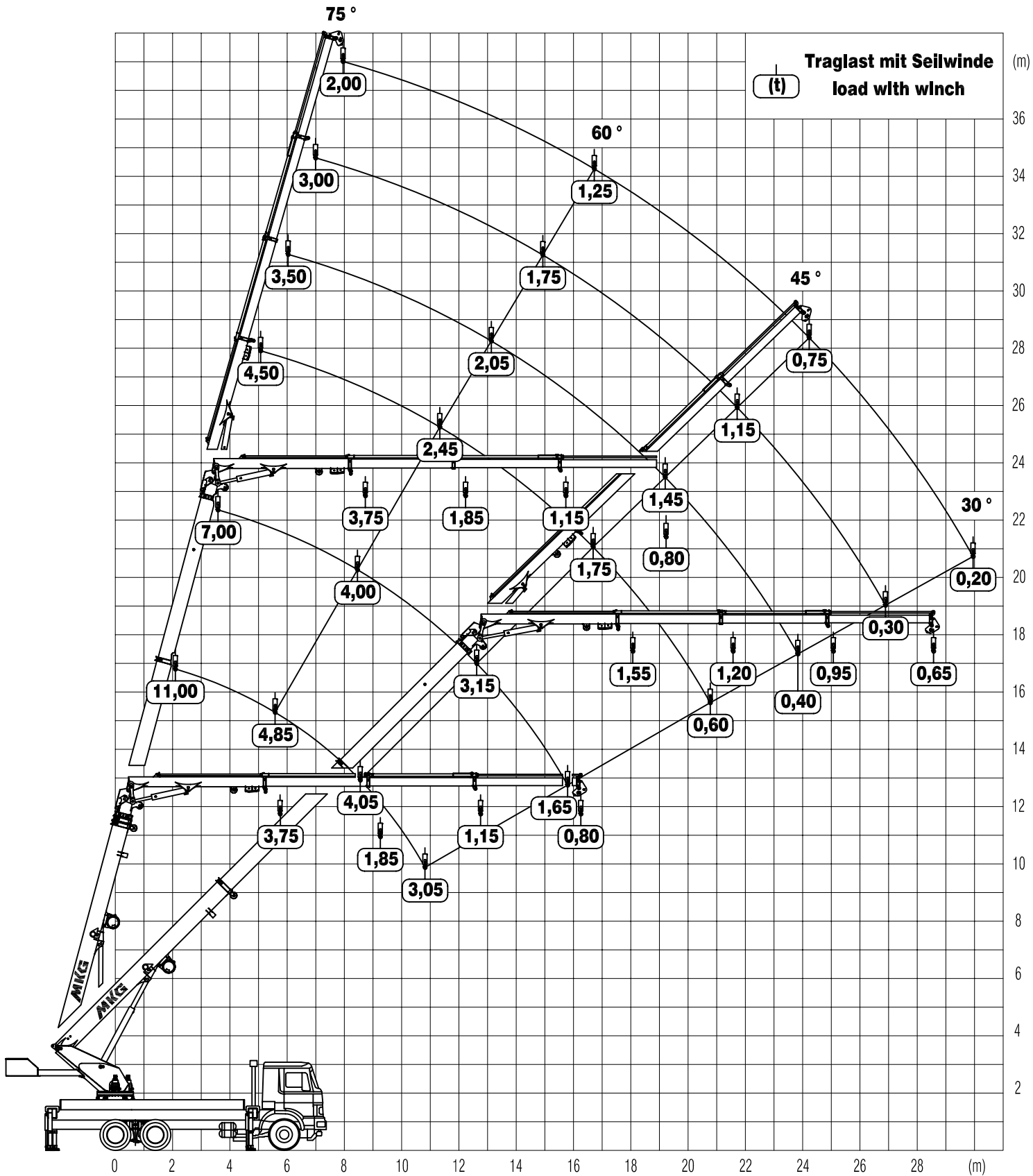
Traglastdiagramm load diagram
