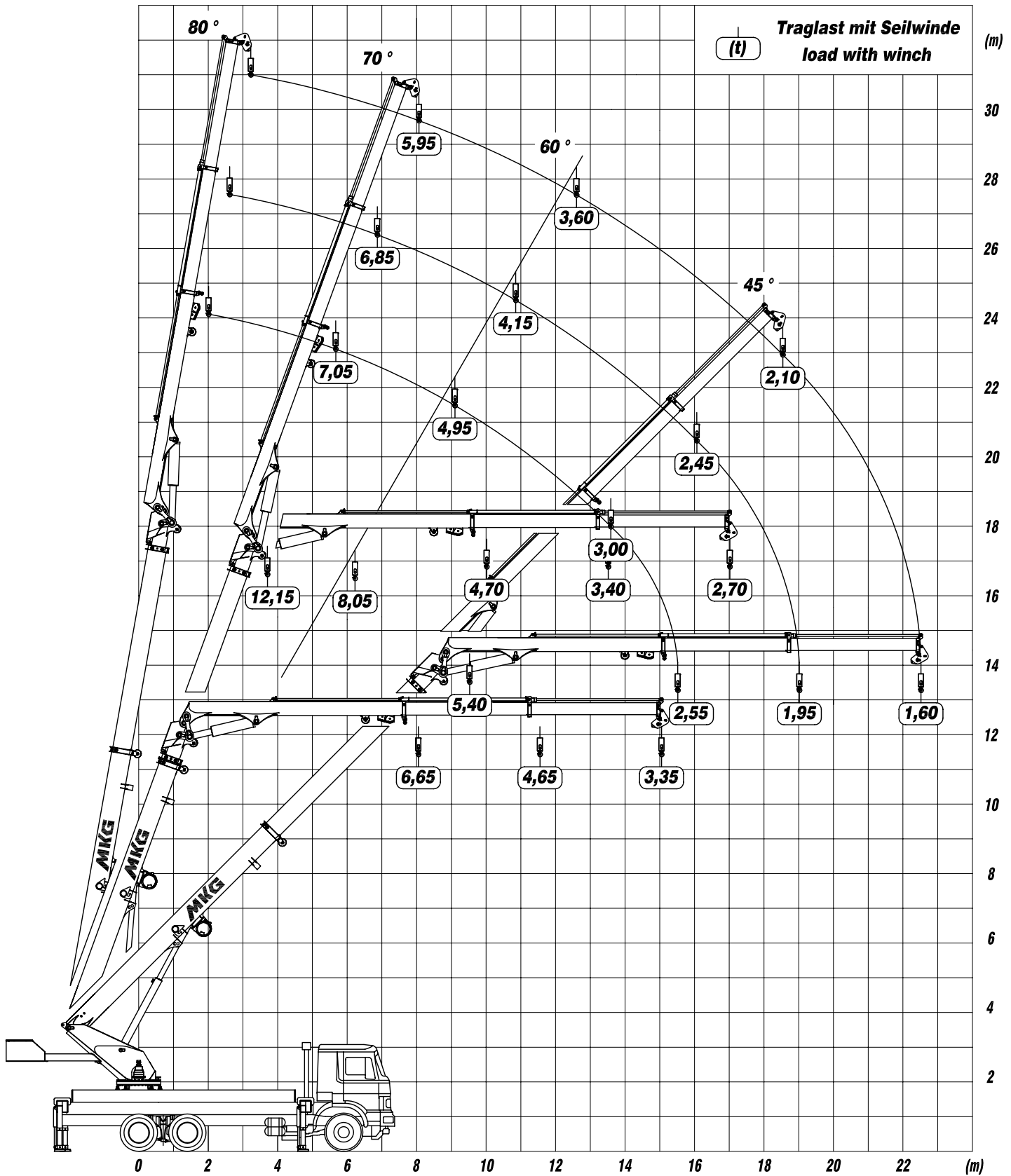
Traglastdiagramm load diagram
