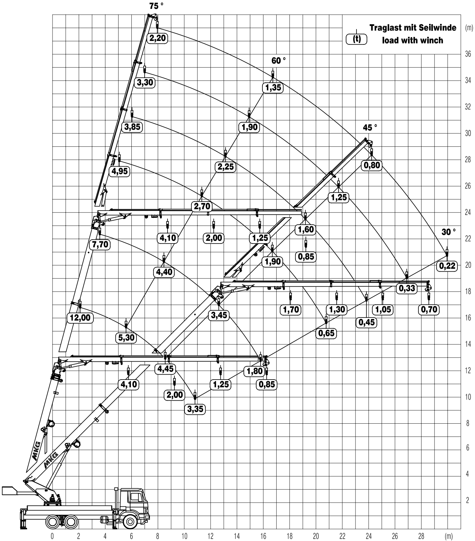
Traglastdiagramm load diagram
